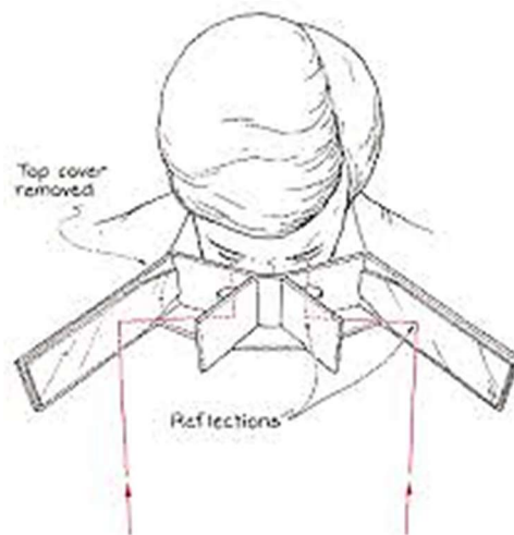
圖三：立體增強鏡(hyperscope)光學結構圖
